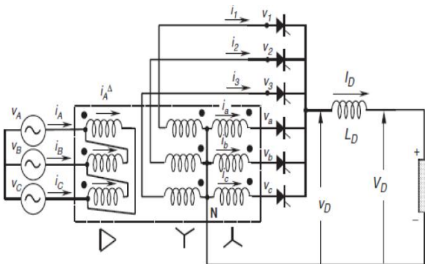
Fig 2: Six-pulse rectifier
